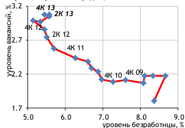
Рисунок 8. Кривая Бевериджа, %
